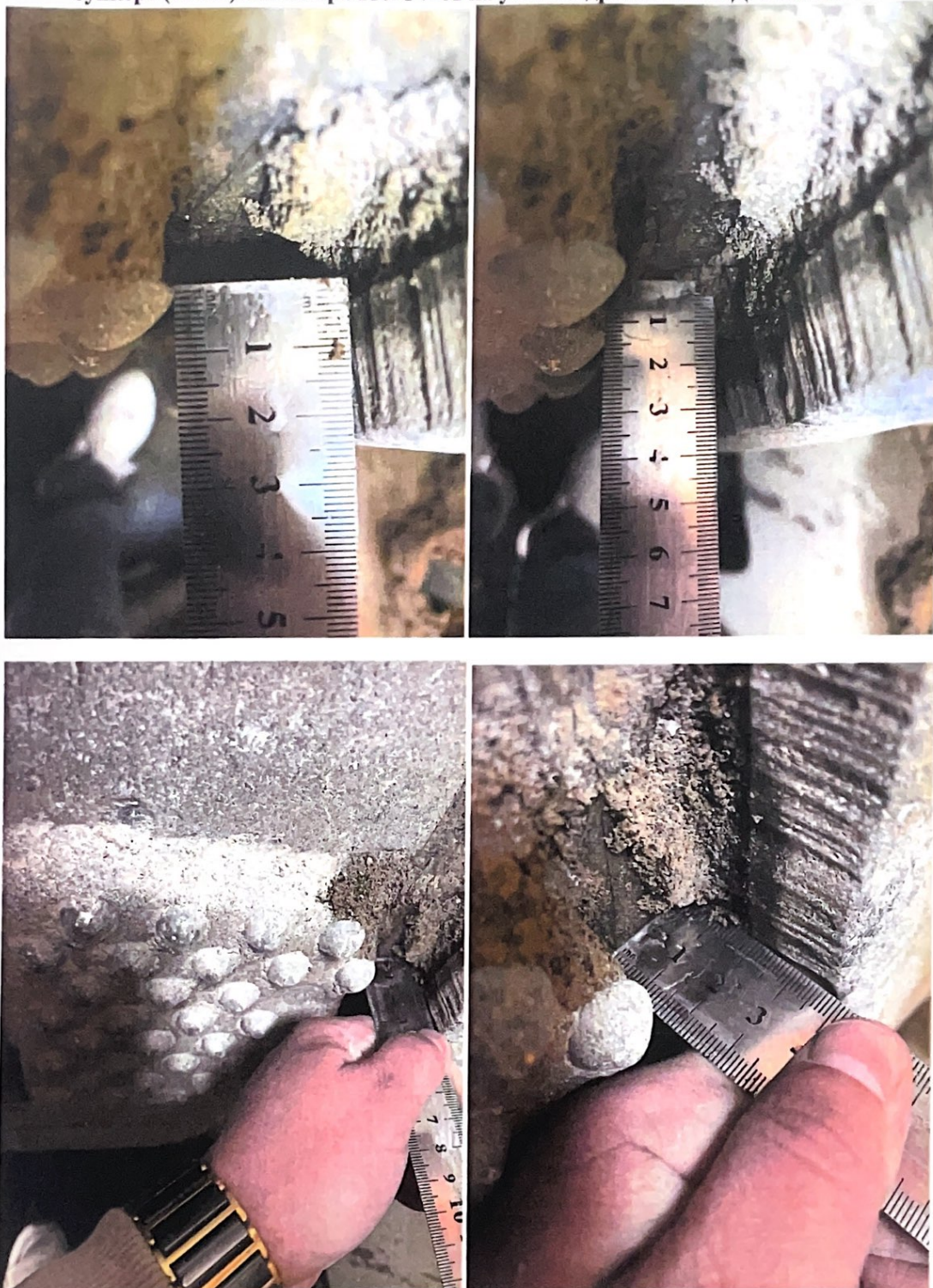
Фото при осмотре модульных пластин BTS Betek установленные на разгрузочном бункере (течка) конвейера 110-CV-01 на участке дробление ККД. 07.10.2024г.
